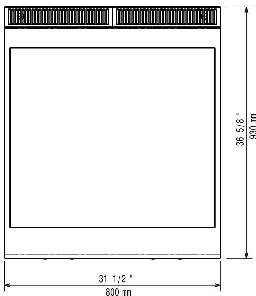
Boven aanzicht
